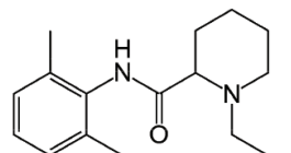
Bupivacaine
