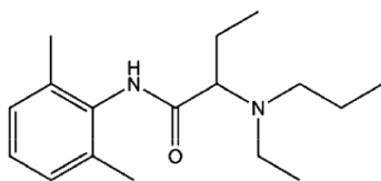
Etidocaine
