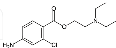
Chlorprocaine
