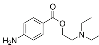
Procaine
