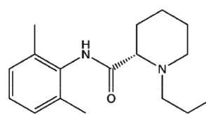
Ropivacaine
