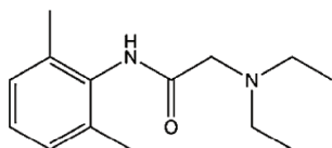
Lidocaine
