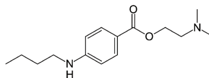
Tetracaine
