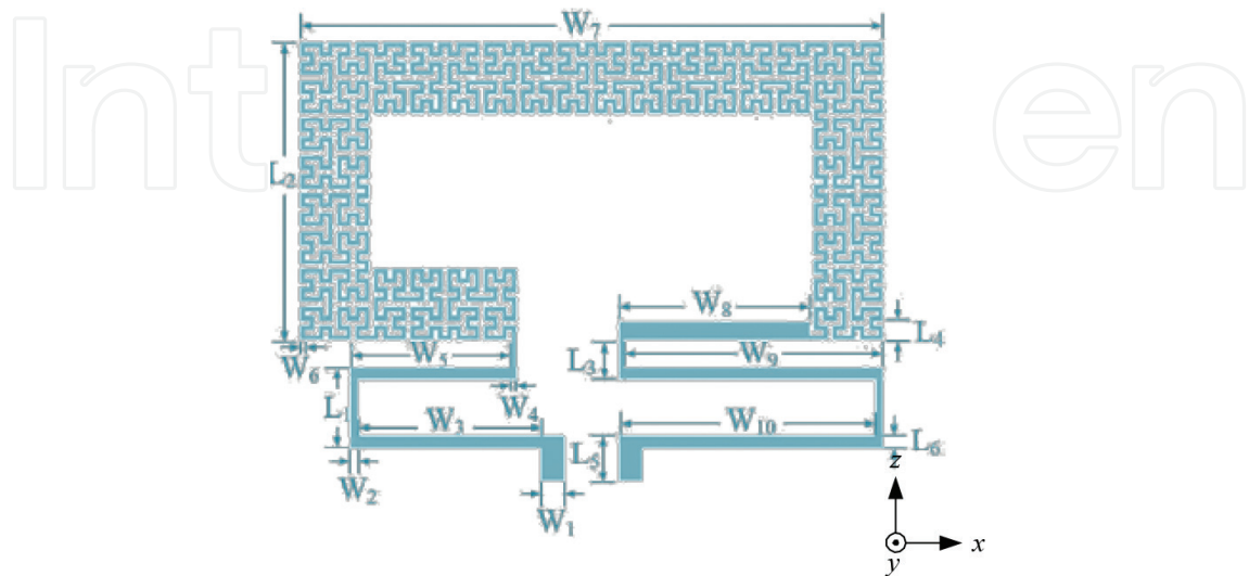
Figure 9. Parameters defining the RFID tag.
