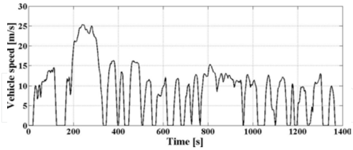
Figure 6. BEV speed (UDDS cycle).
