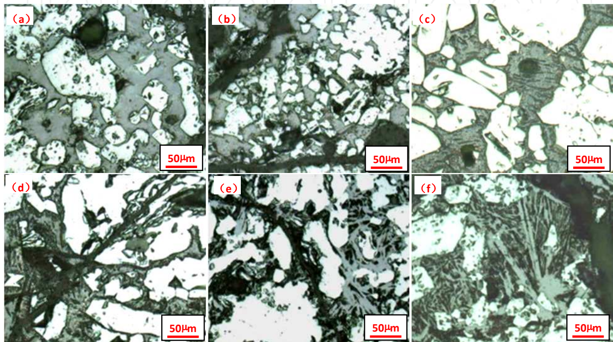
(a) 1280^\circ\text{C} ; (b) 1250^\circ\text{C} ; (c) 1200^\circ\text{C} ; (d) 1150^\circ\text{C} (e) 1050^\circ\text{C} ; (f) Holding 10 min at 1200^\circ\text{C}
