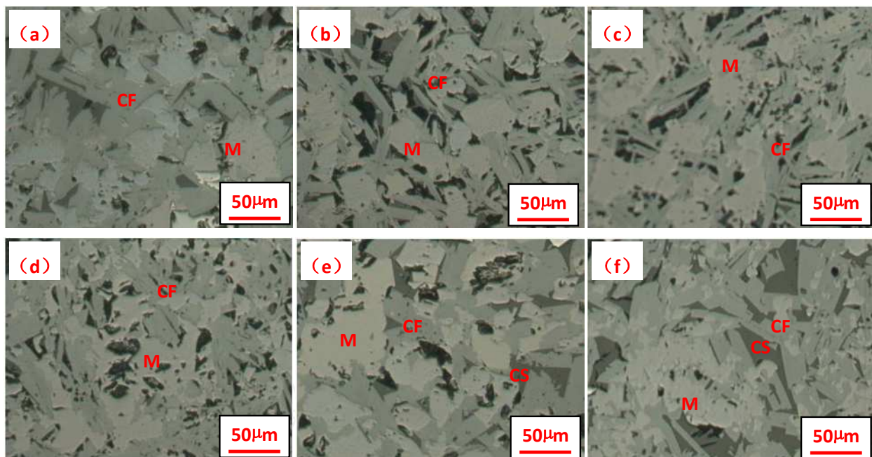
(a) SiO 2 4.3%; (b) SiO 2 4.6%; (c) SiO 2 5.0%; (d) SiO 2 5.4%; (e) SiO 2 5.7%; (f) SiO 2 6.0%
