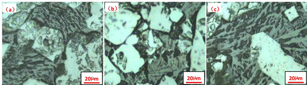
(a) 150°C/min; (b) 100°C/min ; (c) 50°C/min
