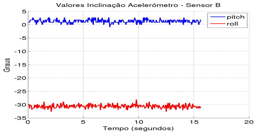
Figura 2.56: Inclinação obtida pelo acelerómetro, com pitch=0^\circ e roll=35^\circ - Sensor B.
