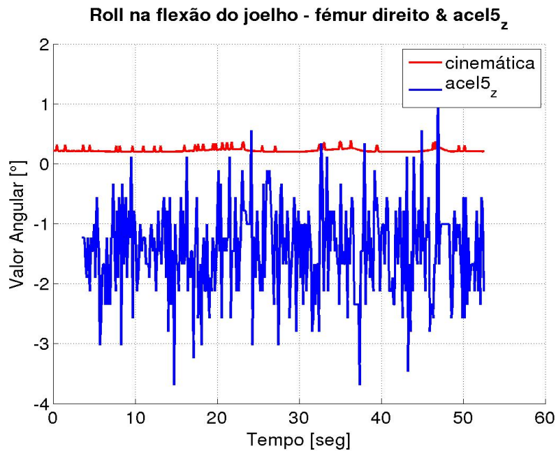
Figura 4.40: Flexão do joelho - fêmur direito - roll obtido através da cinemática e acelerómetro 5.
