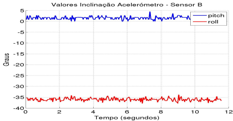
Figura 2.57: Inclinação obtida pelo acelerómetro, com pitch=0^\circ e roll=35^\circ - Sensor B.
