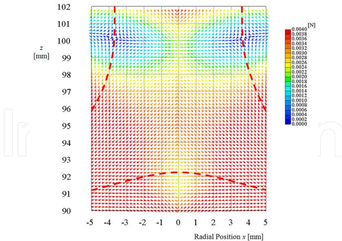
(d) The levitating area when the tilt angle is 1.2^\circ .
