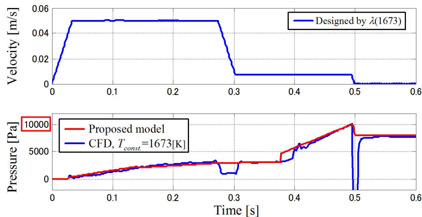
Figure 5. Pressure suppression ( T_{const.}=1673[K] ).
