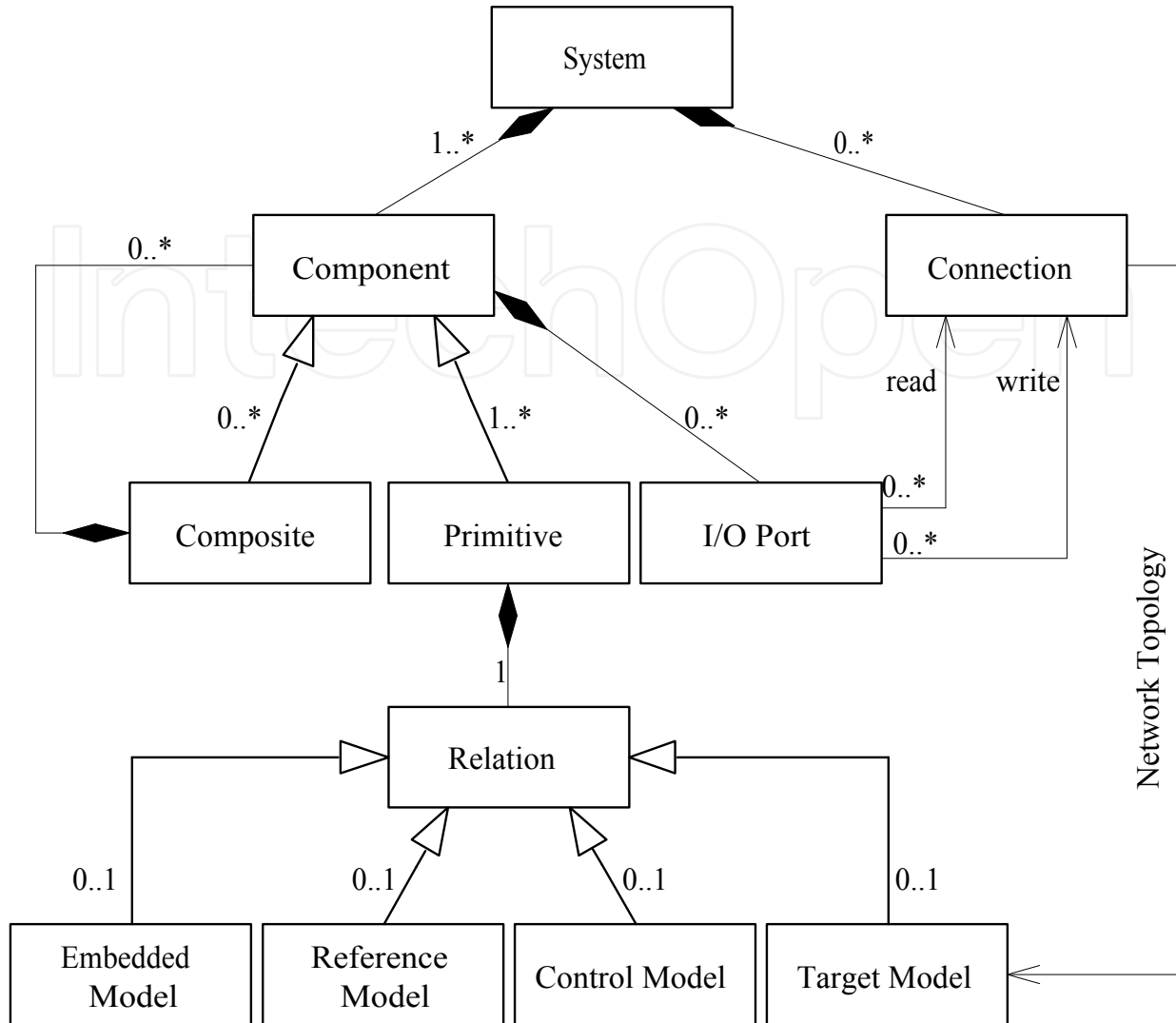
Fig. 2. Framework Meta-Meta-Model
