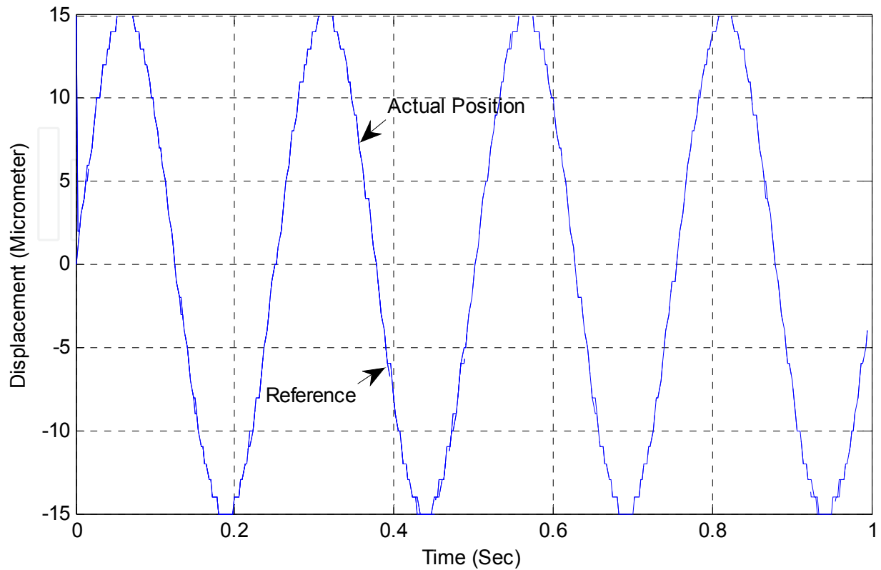
Fig. 2. Desired and Actual Piezoelectric displacement.
