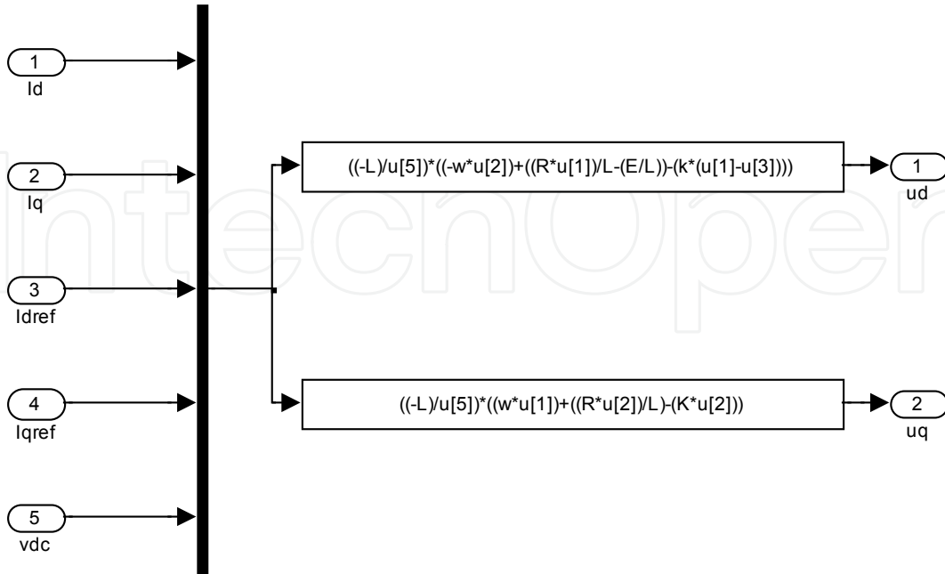
Fig. 12. Input - output controller
