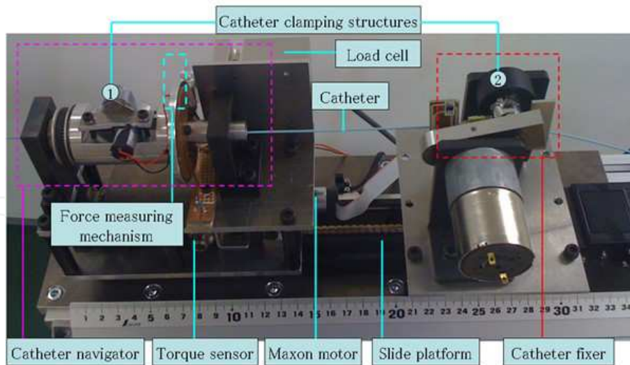
Fig. 22. Slave manipulator
