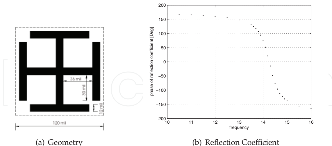
Fig. 10. UC-EBG
