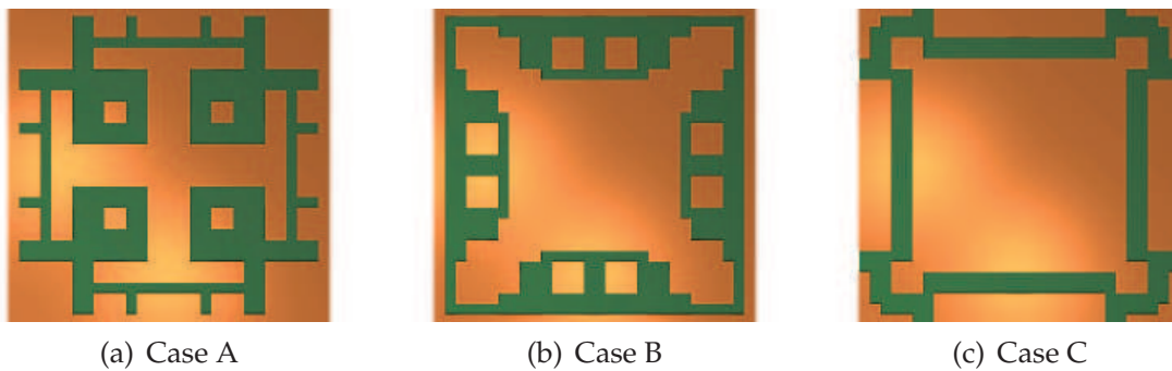
Fig. 14. Best individual
