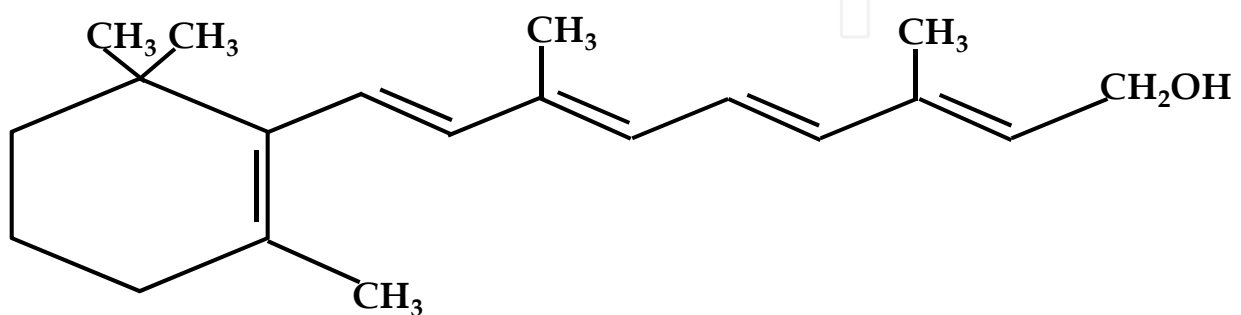
Retinol
