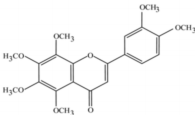
Nobiletin
