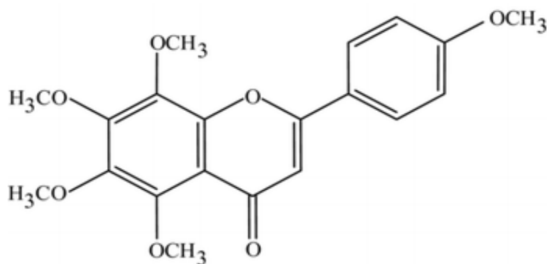
Tangeretin
