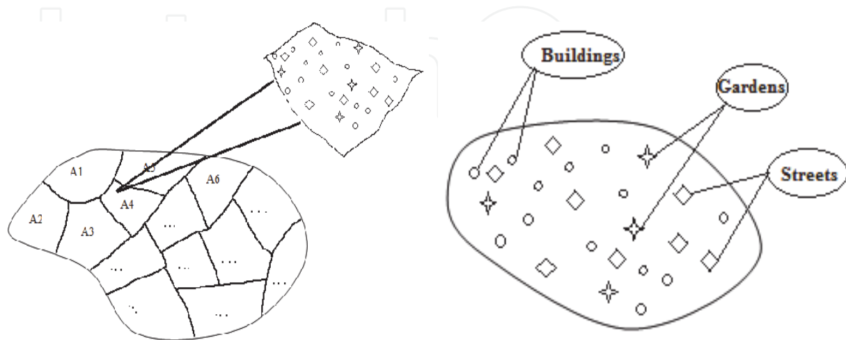
Fig. 14. Space decomposition
