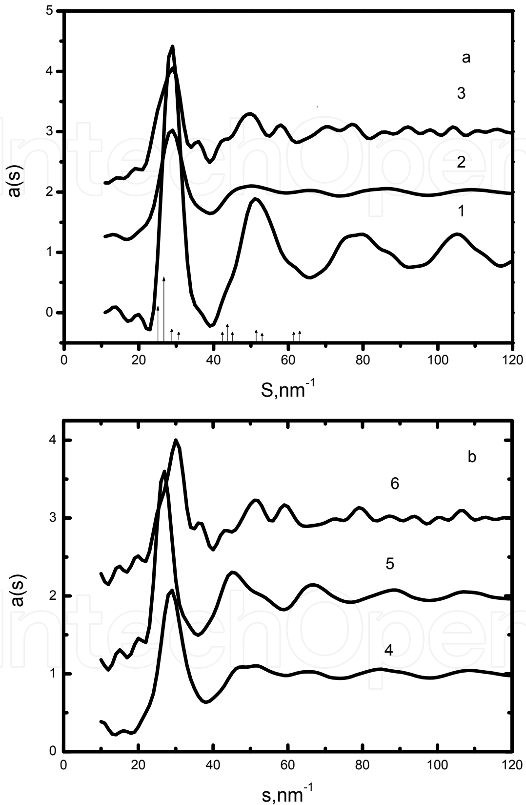
Fig. 10. Amorphous Ni-Zr alloys structure factors with hydrogen and without: a) \text{Ni}_{36}\text{Zr}_{64} (1), \text{Ni}_{36}\text{Zr}_{64}+1\text{H} (2), \text{Ni}_{36}\text{Zr}_{64}+2\text{H} (3); b) \text{Ni}_{64}\text{Zr}_{36} (4), \text{Ni}_{64}\text{Zr}_{36}+1\text{H} (5), \text{Ni}_{64}\text{Zr}_{36}+2\text{H} (6).
