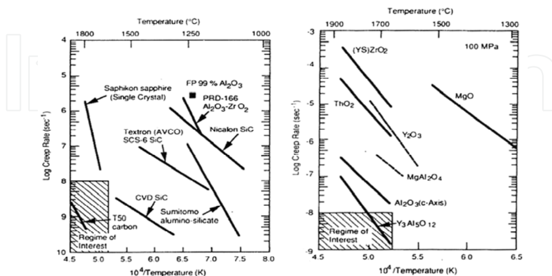
Fig. 24. Creep behaviour
