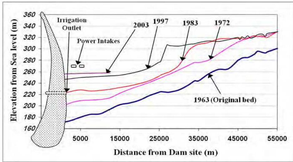
Fig. 6. Sediment longitudinal profile of Dez Reservoir.
