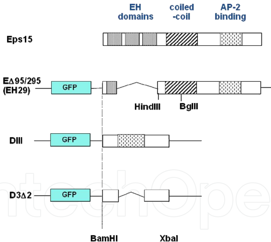
Fig. 1. Eps15 mutants
