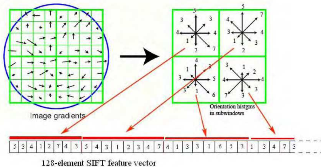
Fig. 9. SIFT Feature Descriptor.
