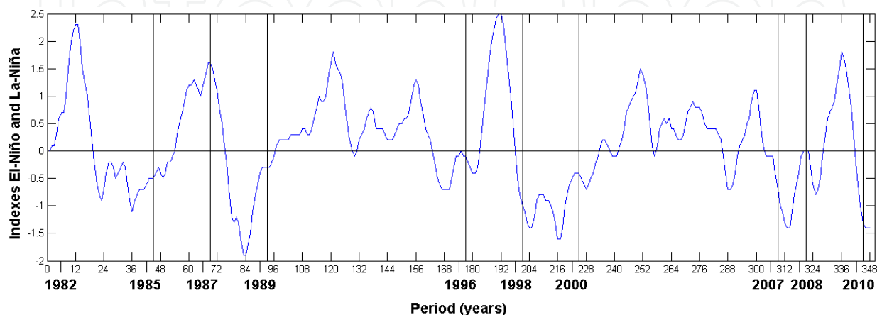
Fig. 6. El Niño and La Niña based in limit of \pm 0.5 °C for the Oceanic Niño Index
