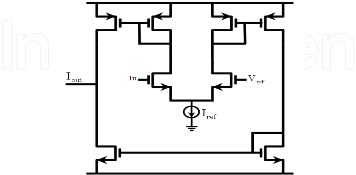
Fig. 9. Mapping circuit.
