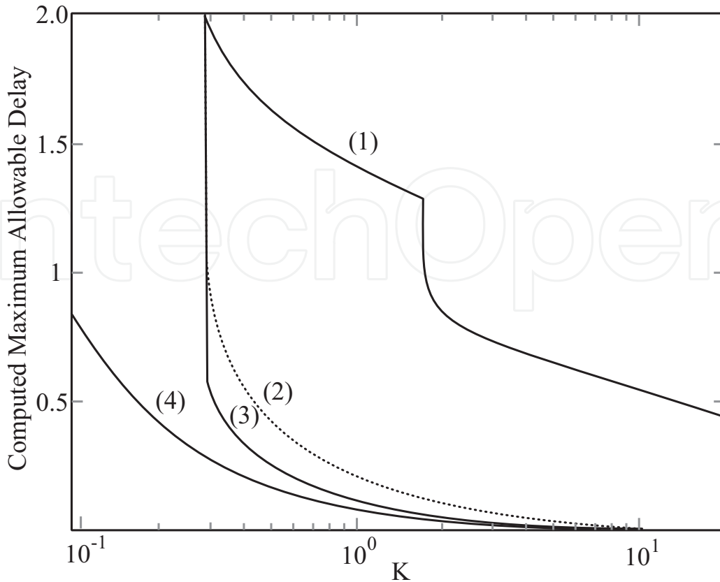
Fig. 5. Delay margin versus K.
