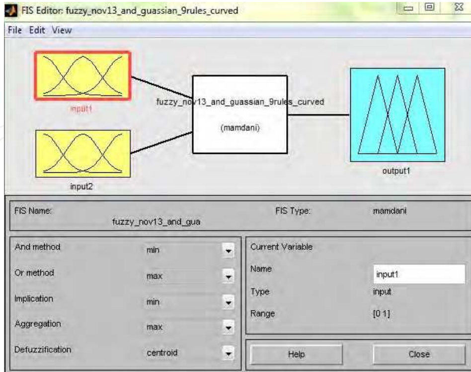
Fig. 6. FIS Model
