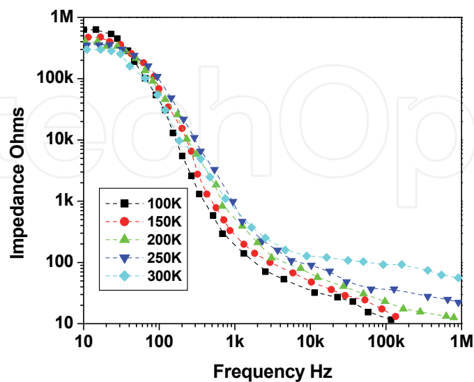
Fig. 15a. Impedance spectra of ITO/PEDOT:PSS/Alq3/Al.
