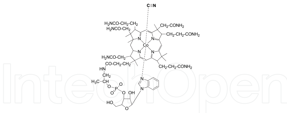
Fig. 11. Vitamine B 12 C 63 H 88 Co N 14 O 14 P.
