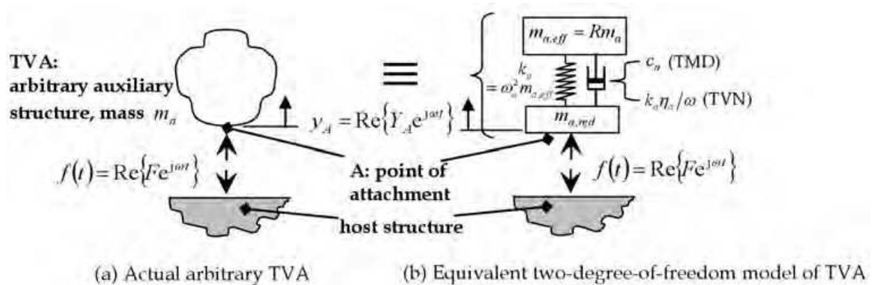
Fig. 1. Generic TVA
