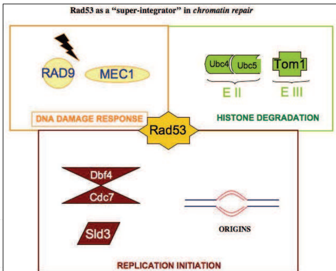
Fig. 3. Rad53 functions
