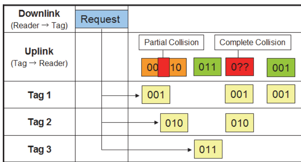
(a) (Pure) ALOHA
