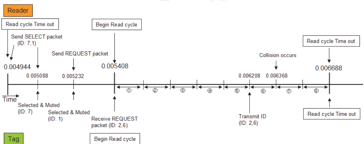
(d) Fourth Read Cycle of the Simulation
