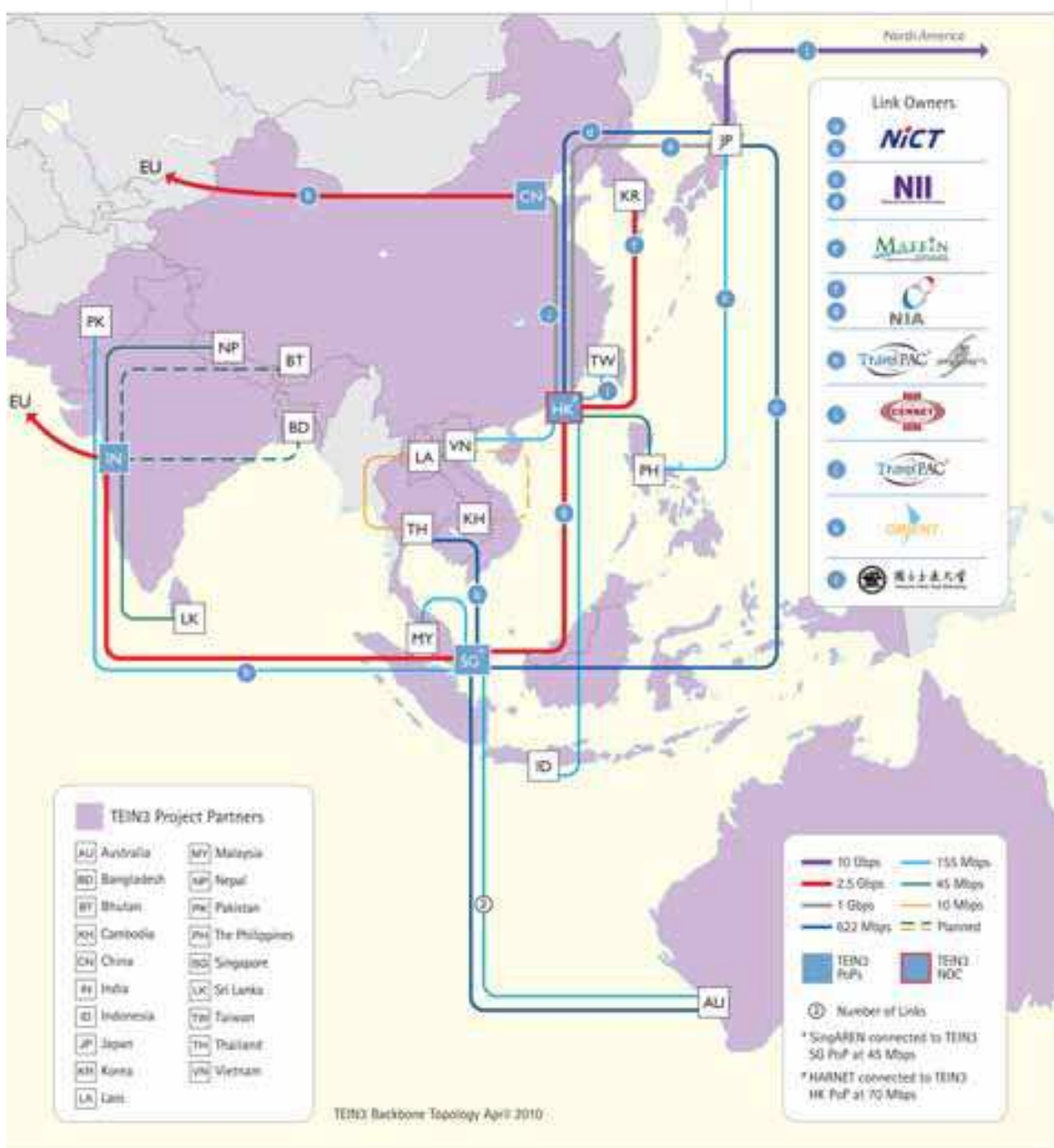
Fig. 7. TEIN3 topology map
