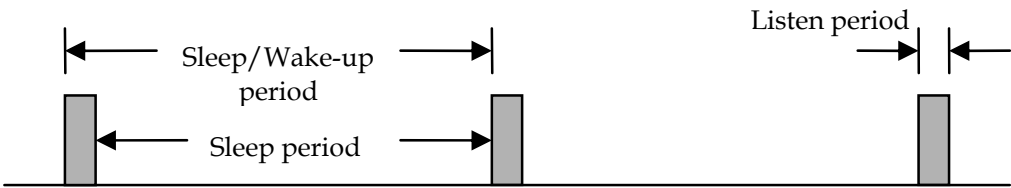
Fig. 1. A periodic wake-up scheme.
