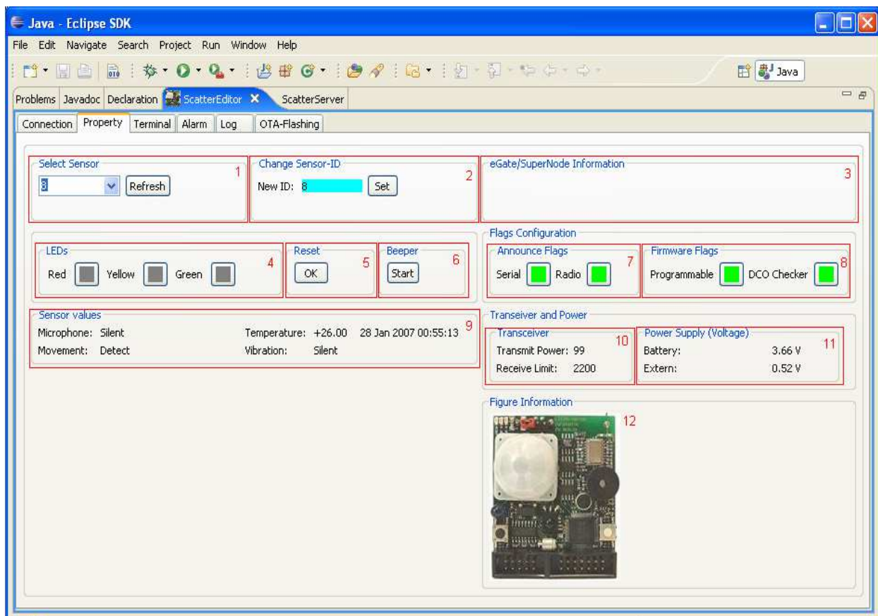
Fig. 16. Property Tabfolder
