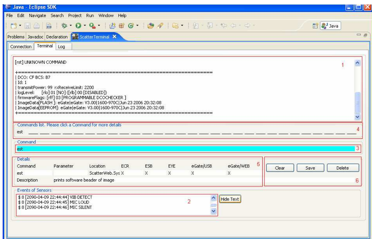
Fig. 17. Terminal Tabfolder
