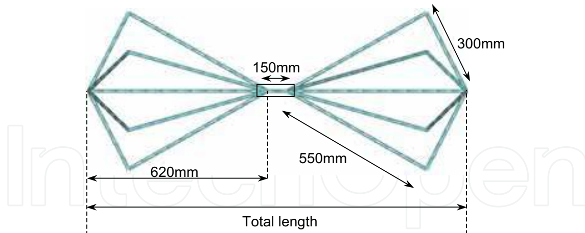
Fig. 19. Test antenna dimensions
