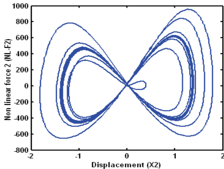
Fig. 6b. (X2, NL-F2) "Van Der Pol case"
