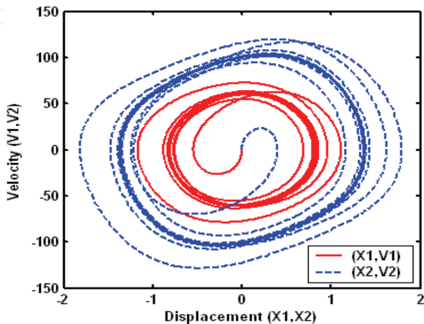
Fig. 5b. Phase diagrams "Van Der Pol case"
