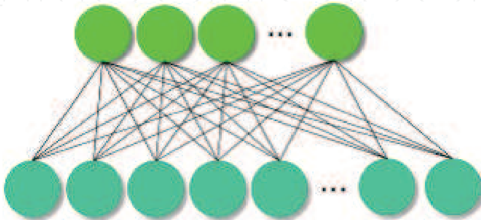
Fig. 7. Supervised SOM
