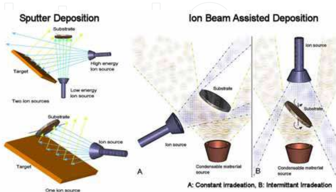
Fig. n.4. Deposition Configuration
