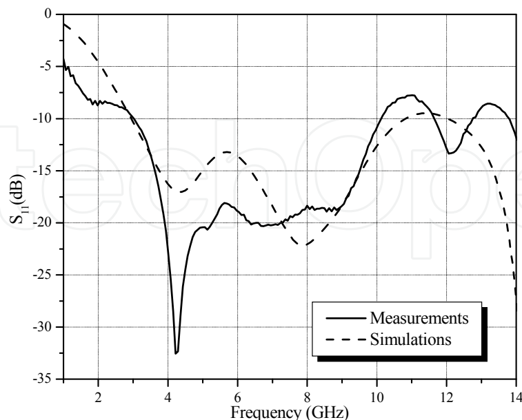
Fig. 22. Antenna return loss
