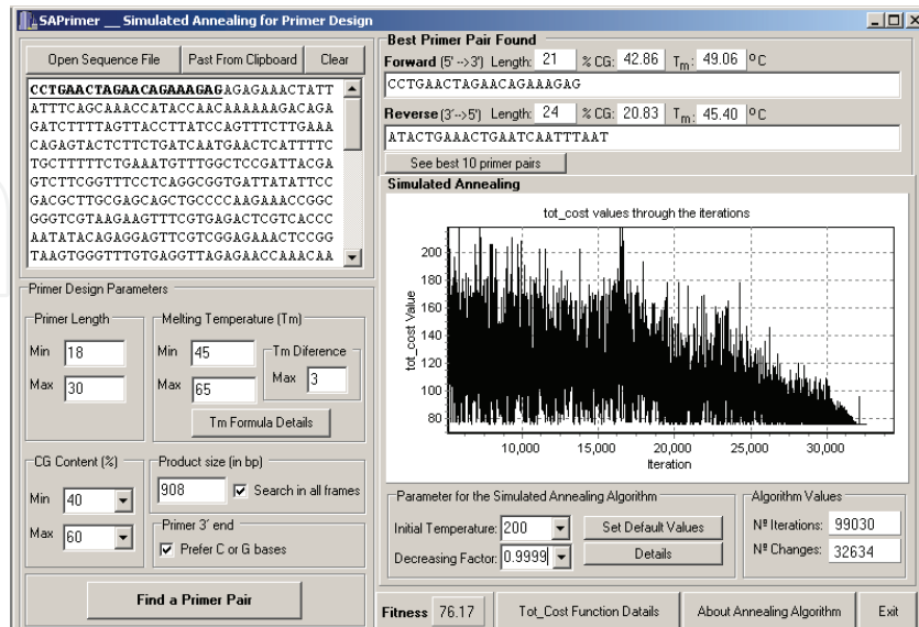
Fig. 4. SAPrimer (R2) interface
