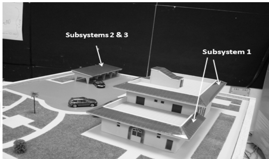
Fig. 17. Villa prototype
