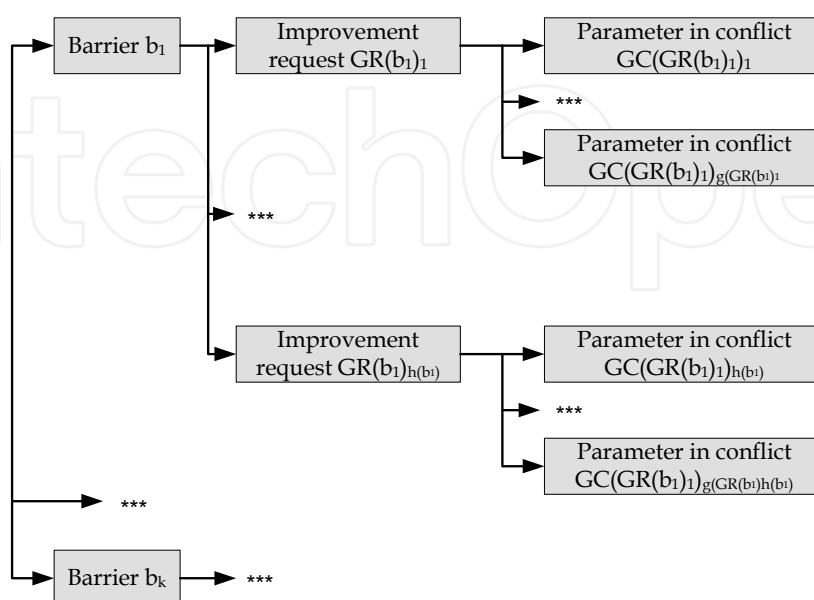
Fig. 3. Step 3 of Sigma-TRIZ
