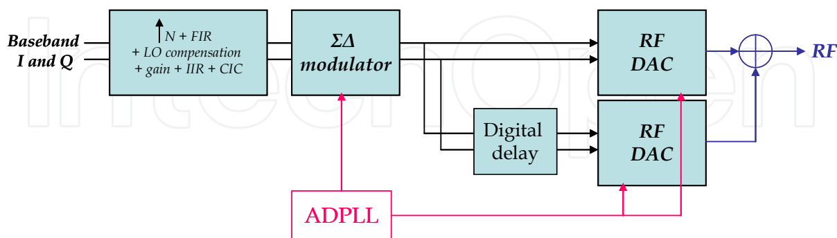
Fig. 22. Sigma Delta - RF-DAC architecture [Pozsgay et al]
