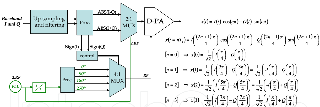
Fig. 23. Digital Quadrature Modulator [Parikh et al]
