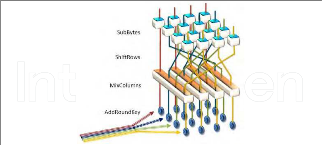
Fig. 3. AES Round
