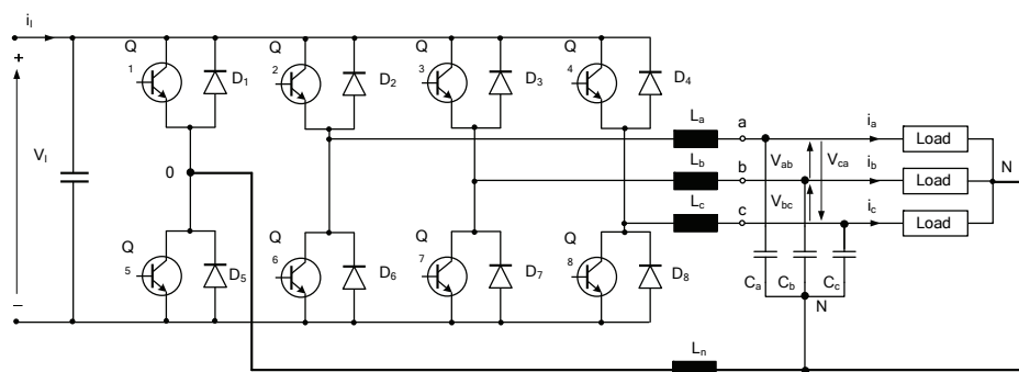
Fig. 21. Four-leg inverter.
