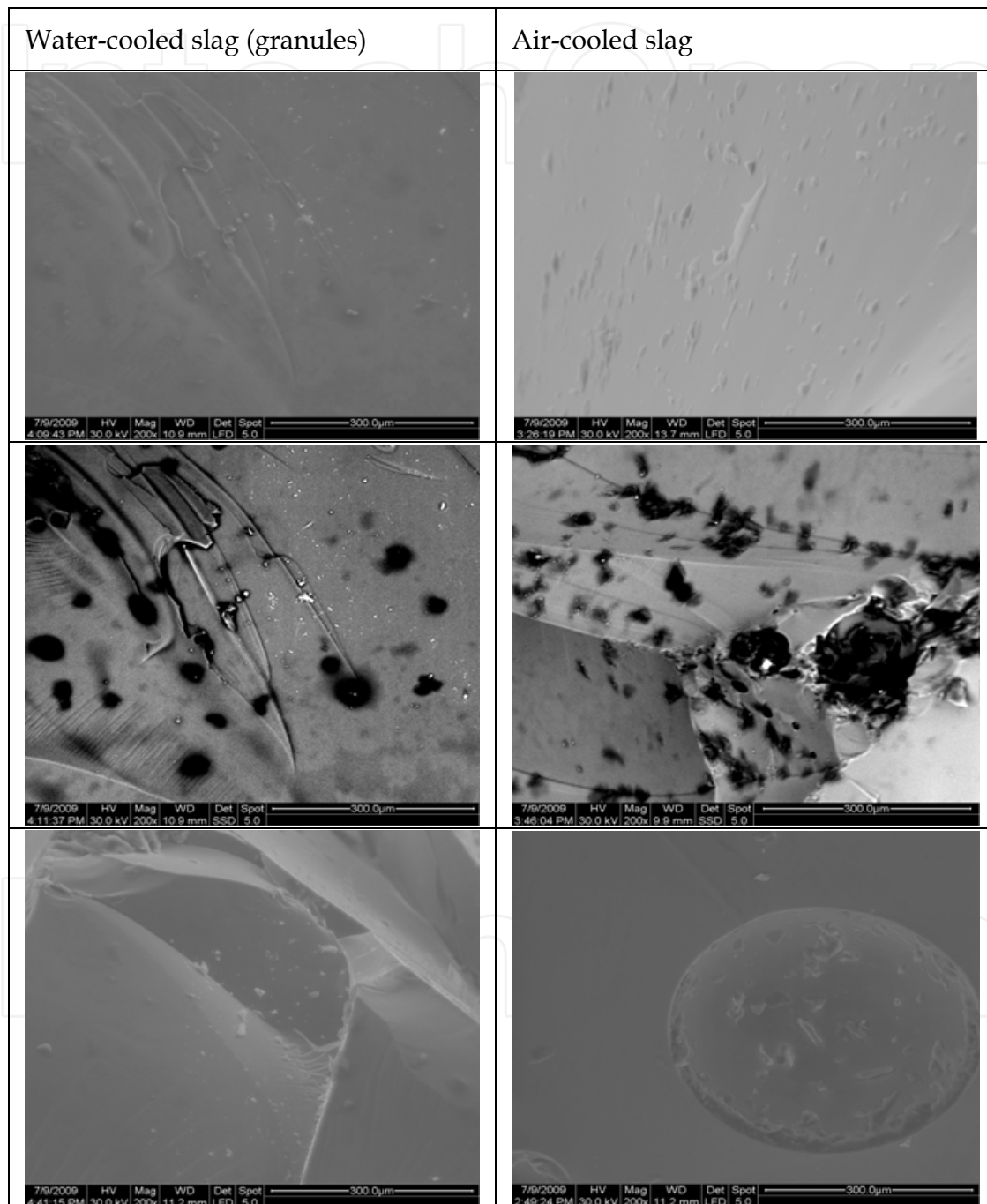
Fig. 20. SEM images
