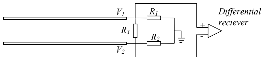
a. Pi-termination
