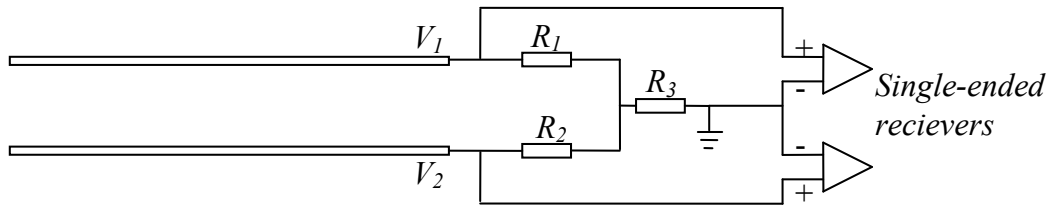
b. T-termination
