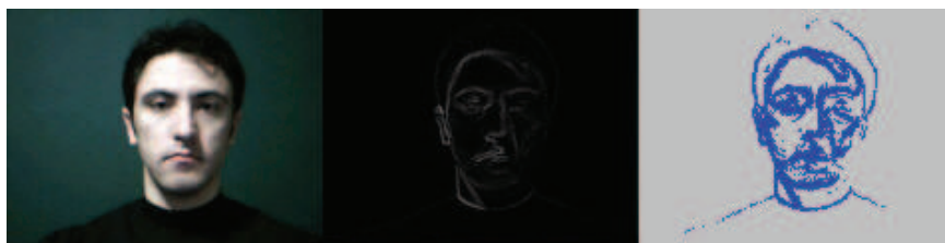
Fig. 5. Edge detection
