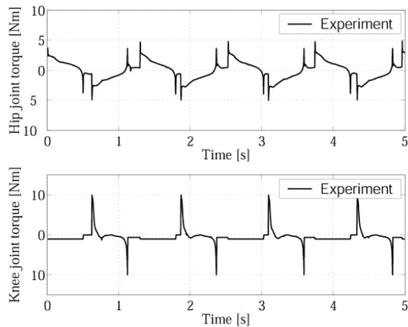
Fig.19. Joint input torque (Hase T. & Huang, Q., 2005).
