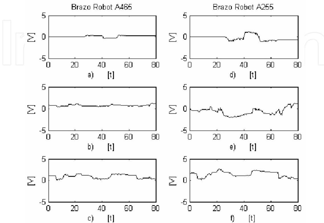
Fig. 8. Input voltages. a) v_{11} . b) v_{12} . c) v_{13} . d) v_{21} . e) v_{22} . f) v_{23} . ---- experiment - - - simulation.
