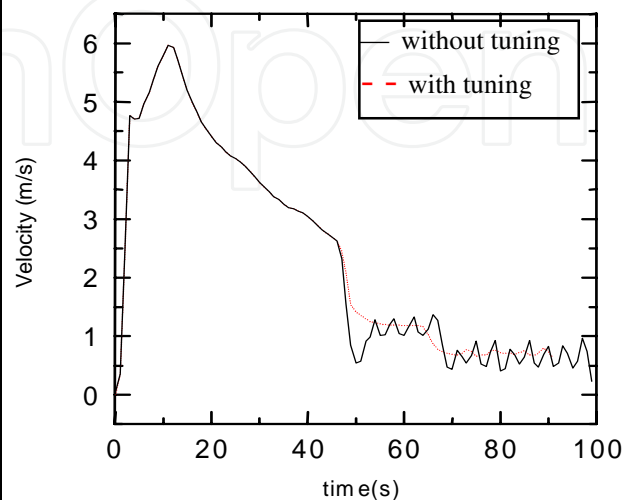
Fig. 27. Velocity Profiles.
