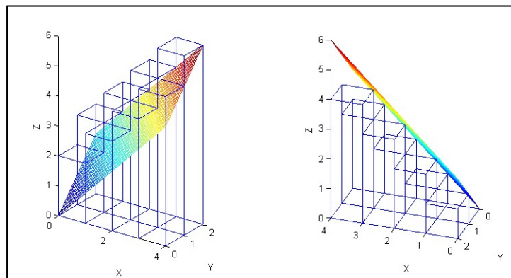
Figura 3: Particiones para obtener la Suma superior y suma inferior de f(x, y) = x + y .
